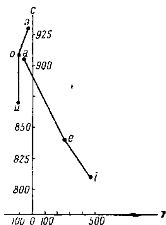
Схема 10. График зависимости C = f(T) для армянских гласных.
