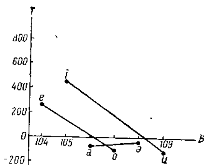
Схема 11. График зависимости T = f(b) для армянских гласных.
