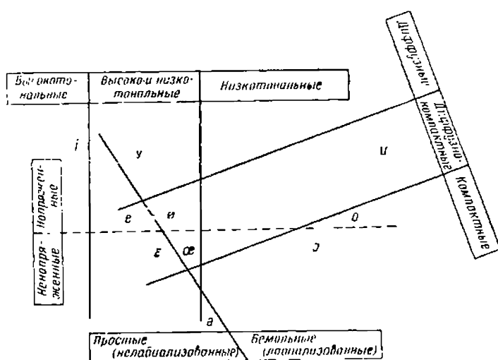
Схема 17. Акустическая (спектральная) параметризация системы французских гласных.
