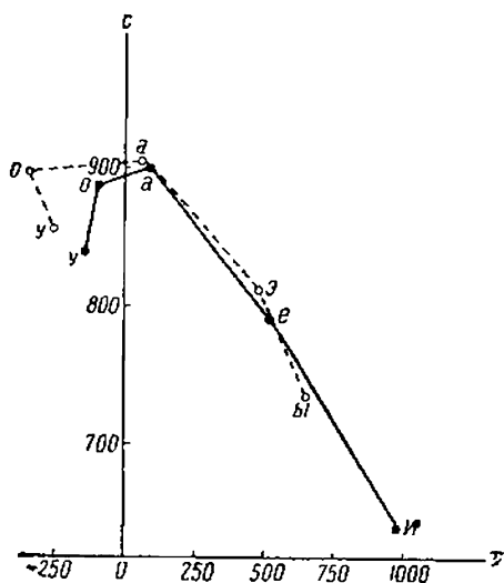
Схема 7. График зависимости C = f(T) для русских гласных (по данным Халле — фонологическая модель Трубецкого — Авапесова): \circ — позиции гласных, стоящих после [n] , \bullet — позиции гласных, стоящих после [n'] .
