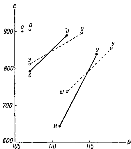
Схема 6. График зависимости C = f(b) для русских гласных (по данным Халле — фонологическая модель Трубецкого — Авапесова): \circ — позиции гласных, стоящих после [n] , \bullet — позиции гласных, стоящих после [n'] .
