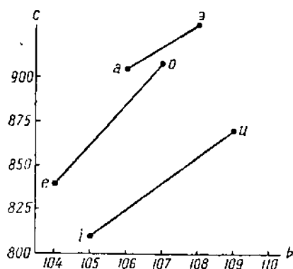
Схема 9. График зависимости C = f(b) для арийских гласных.
