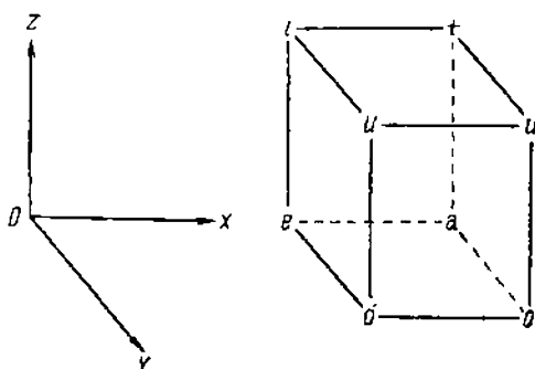
Схема 4. Функционально-семиотическая параметризация системы турецких гласных фонем*
