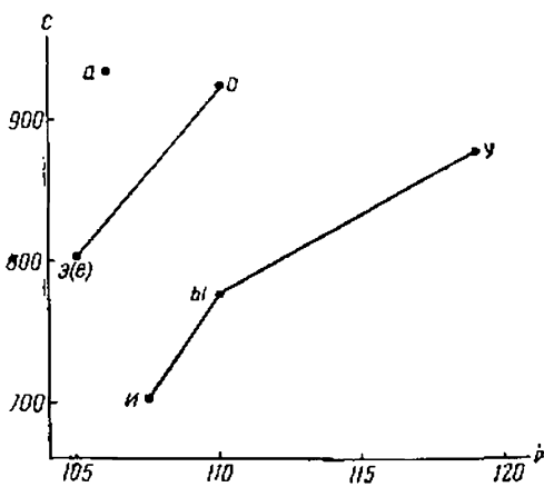
Схема 5. График зависимости C = f(b) для русских гласных (по данным Фанта — фонологическая модель Шербы)
