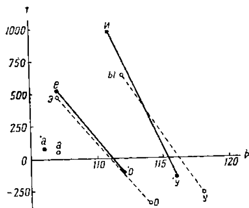
Схема 8. График зависимости T = f(b) для русских гласных (по данным Халле-фонологическая модель Трубского — Аванесова): ○ — позиции гласных, стоящих после [и], ● — позиции гласных, стоящих после [п'].
